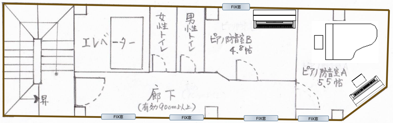
2F
